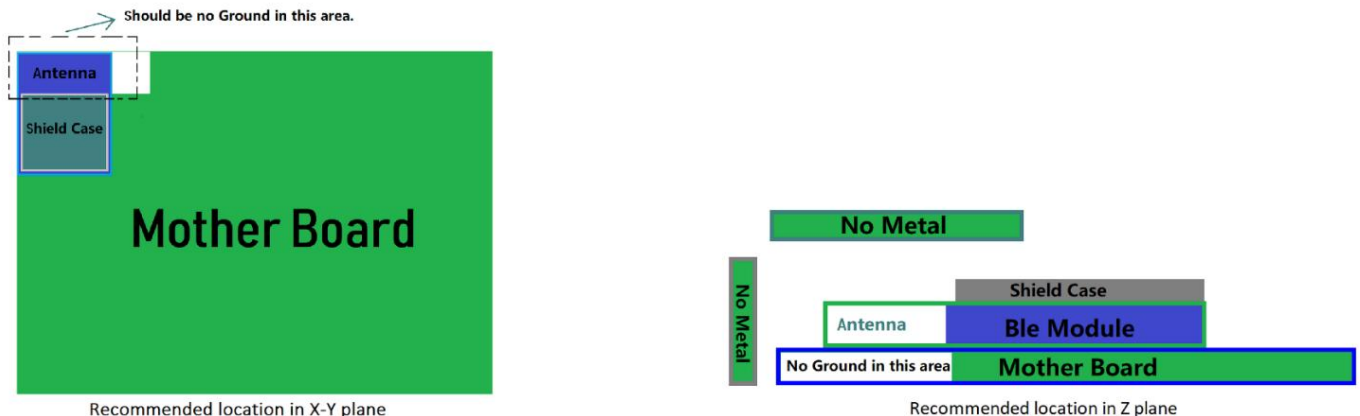
图 3-模块布局参考示意图
