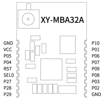
图 1-模块引脚图
